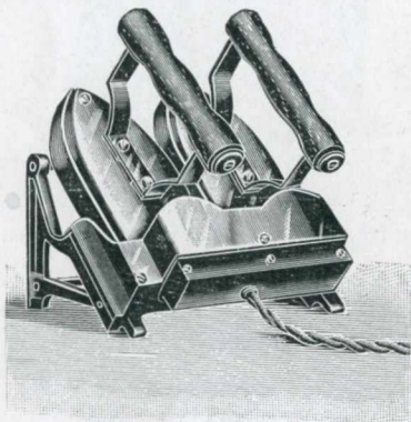
N° 120. Support prise de courant avec 2 fers n° 116.
